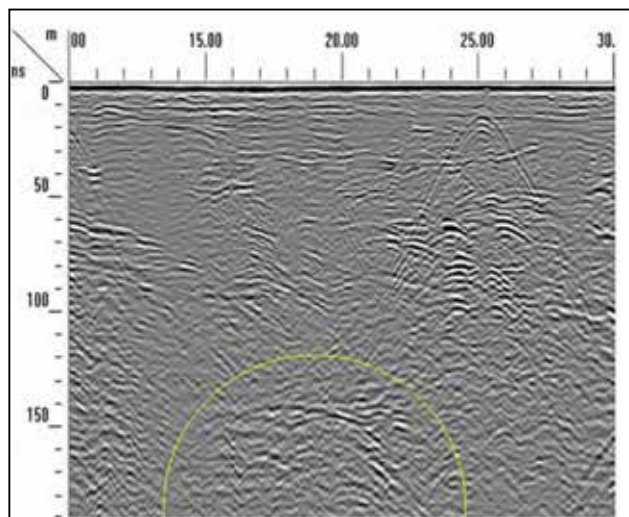
Dati UtilityScan utilizzando la tecnologia HyperStacking
