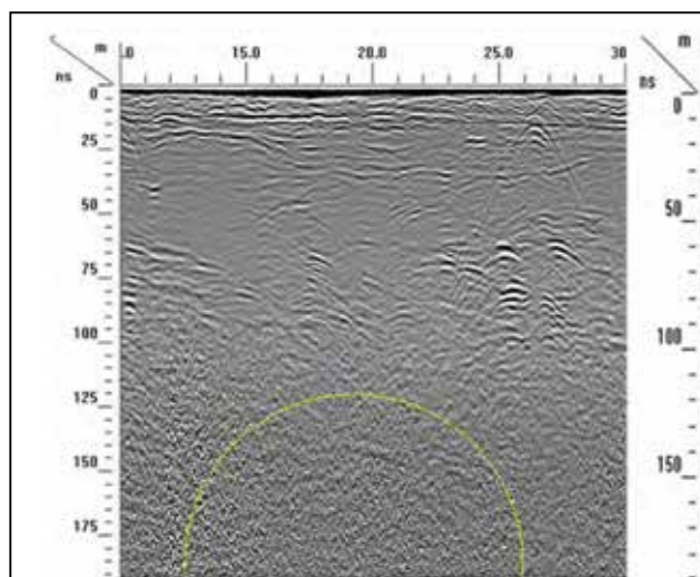
Dati raccolti con la tecnologia GPR Standard
